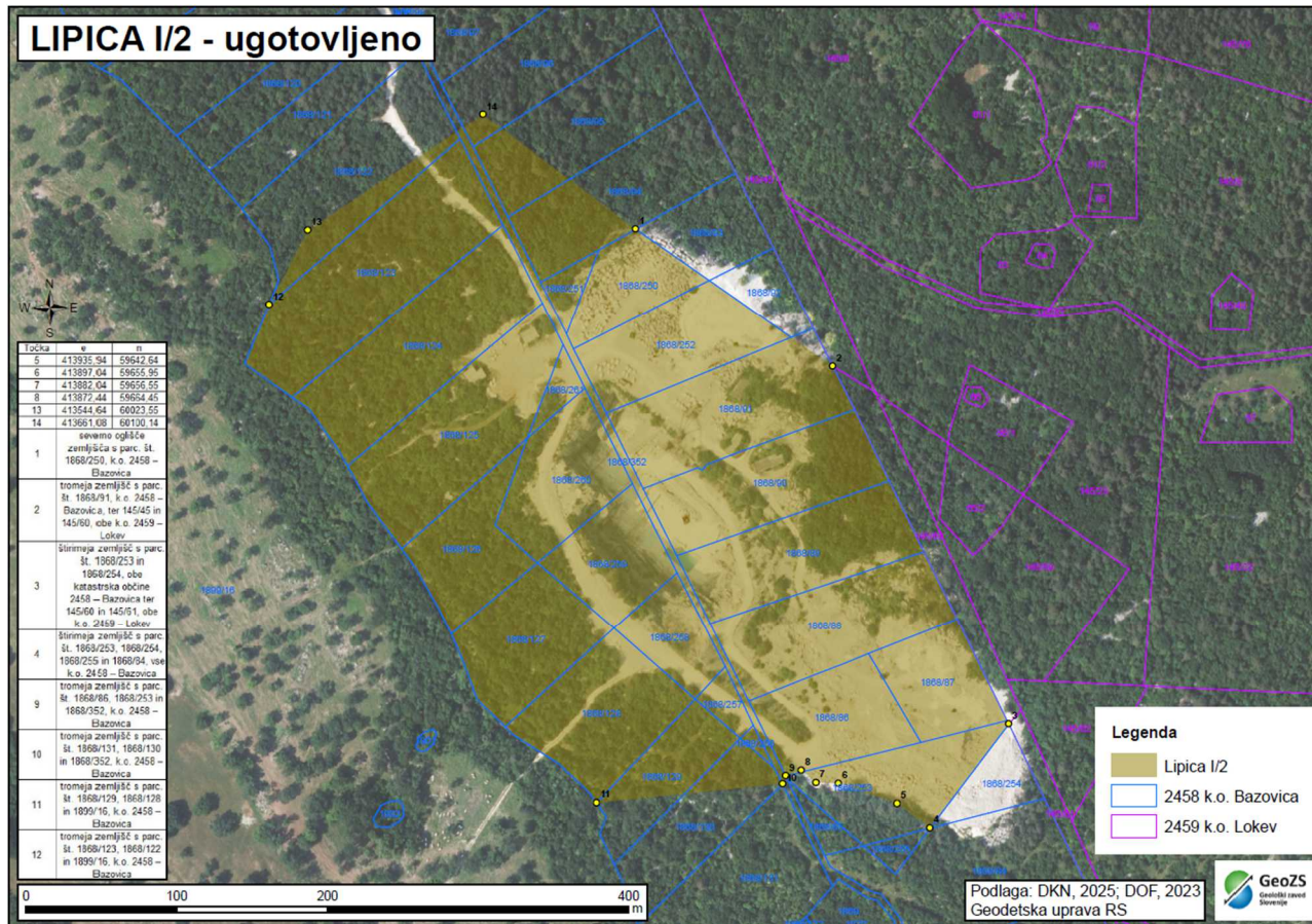
Slika 2: Situacijski načrt pridobivalnega prostora Lipica I/2 na katastrski in topografski podlagi
