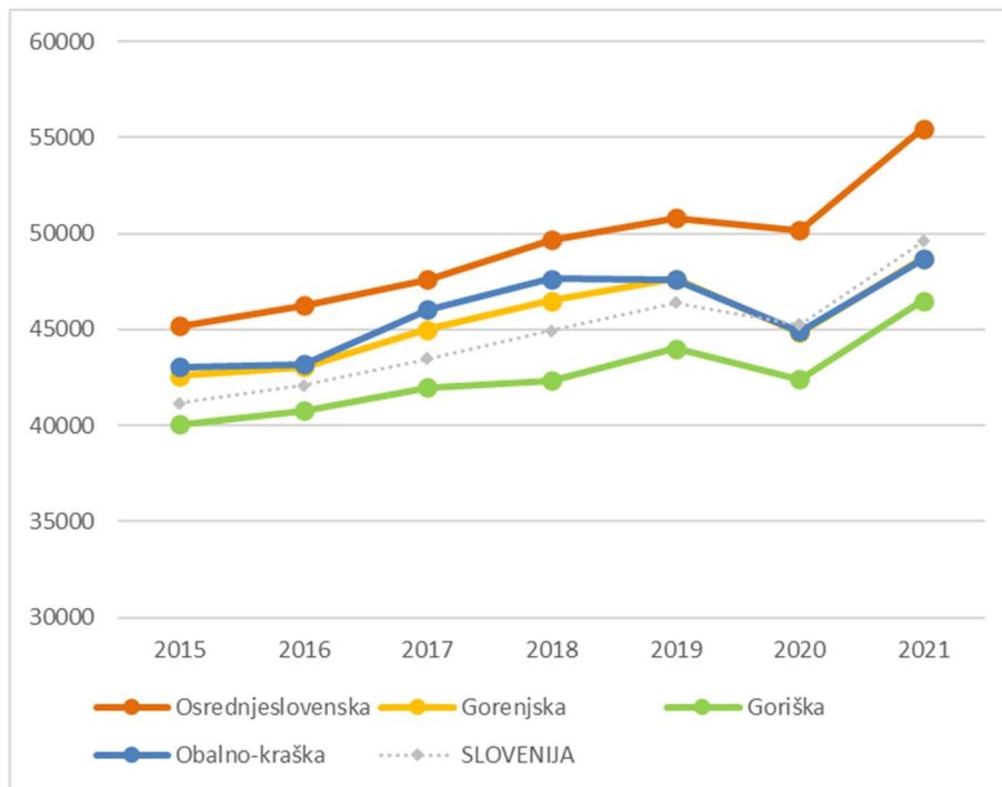
Slika 8: BDP na zaposlenega v razvojnih regijah, ki so del KRZS (v evrih)
