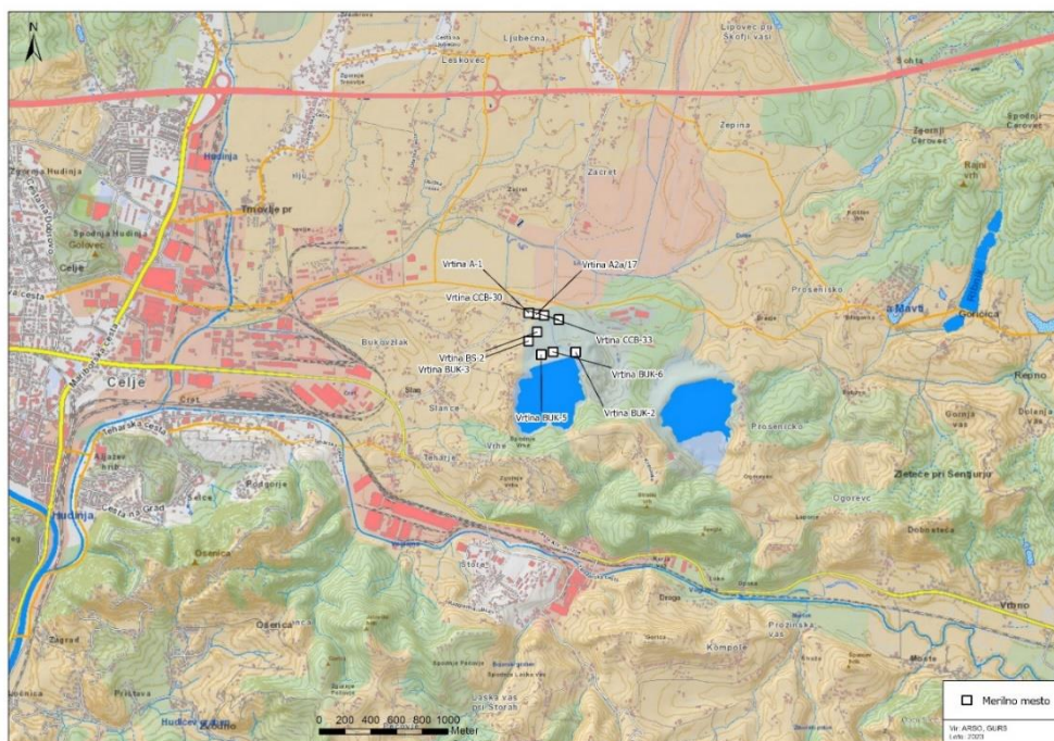
Slika 6: Merilna mreža (lokacije piezometrov) na odlagališču Bukovžlak
