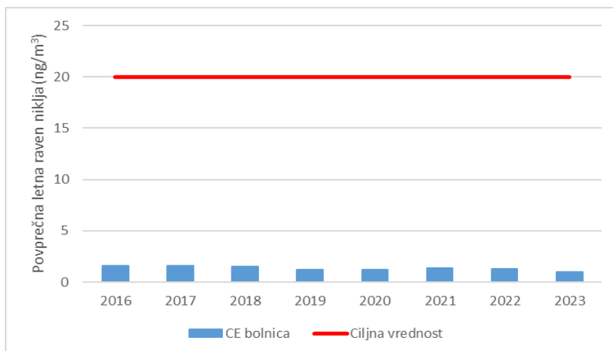
Grafikon 7: Povprečne letne ravni niklja v obdobju 2016–2023; ravni so podane v \text{ng/m}^3 .
