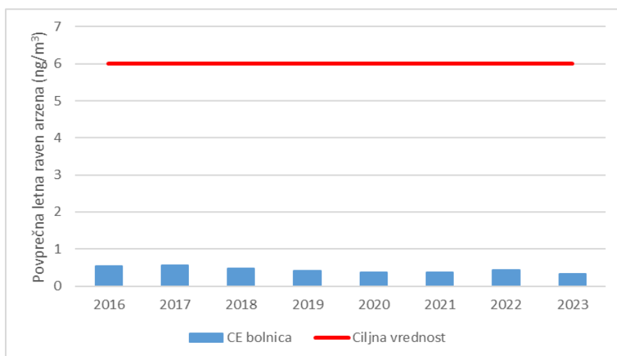
Grafikon 5: Povprečne letne ravni arzena v obdobju 2016–2023; ravni so podane v ng/m³.
