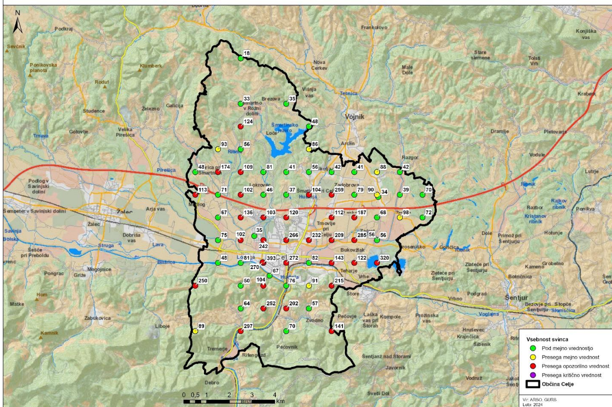
Prostorski prikaz vsebnosti svinca (mg/kg suhe snovi) v tleh Mestne občine Celje
