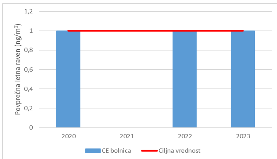
Grafikon 4: Povprečne letne ravni benzo(a)pirena v letih 2020, 2022 in 2023; ravni so podane v ng/m³.
