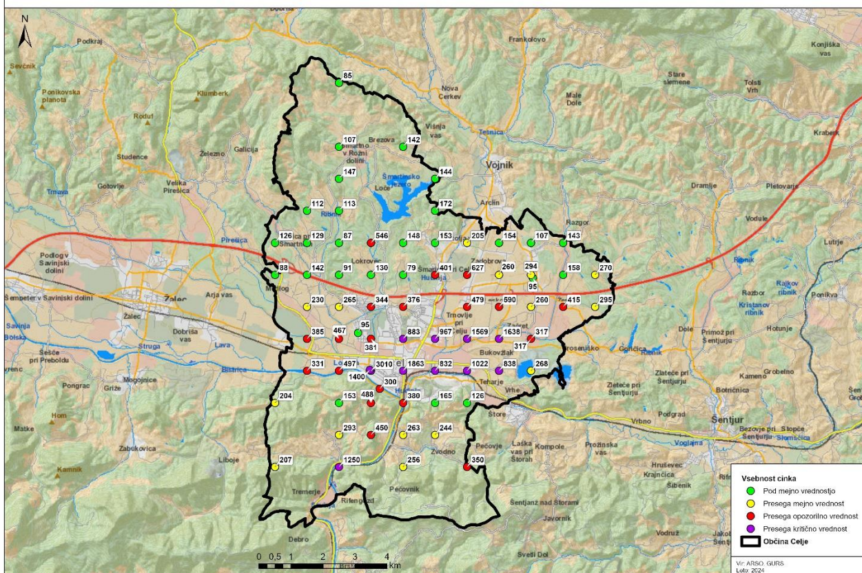
Prostorski prikaz vsebnosti cinka (mg/kg suhe snovi) v tleh Mestne občine Celje
