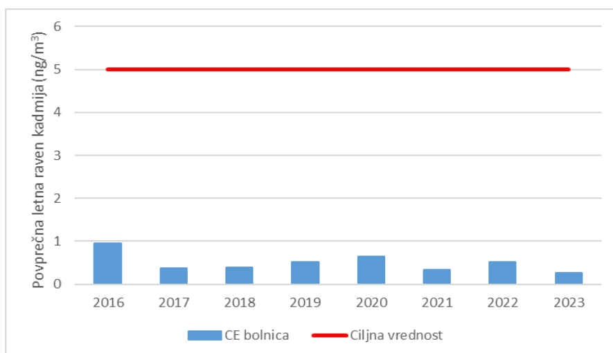
Grafikon 6: Povprečne letne ravni kadmija v obdobju 2016–2023; ravni so podane v ng/m³.
