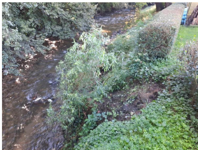
Zajede brežin in poškodovano obrežno zavarovanje ob hiši Dobrava pri Konjicah 4E
